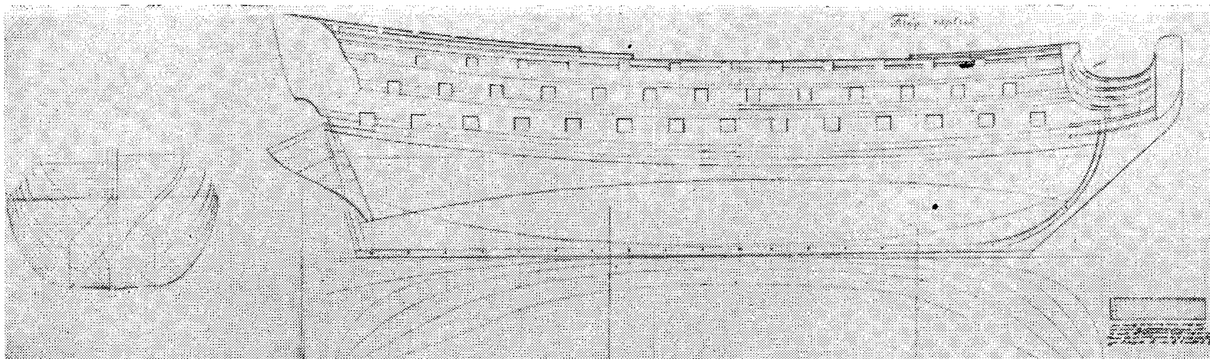
Рис. 3. Чертеж 100-пушечного корабля «Петр» (ф. 327, оп. 1, д. 482).
